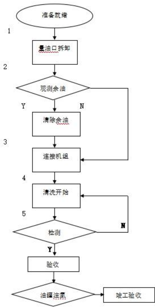
图 2.7-1 清罐流程图
