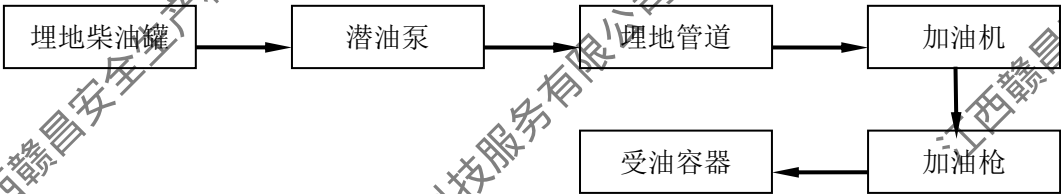
图 2.5-4 柴油加油工艺流程图示意图
