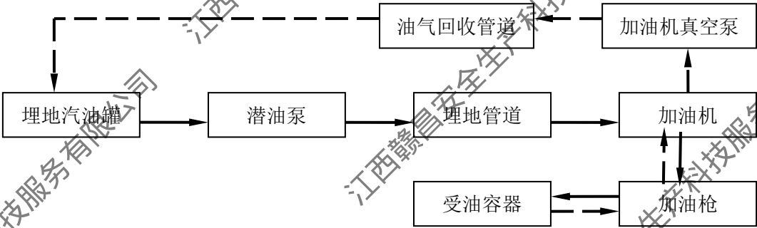
图 2.5-3 汽油加油工艺流程图示意图
